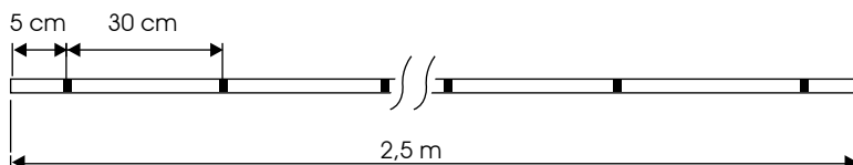
Figura 78 – Esquema de colocação dos parafusos no perfil de arranque
