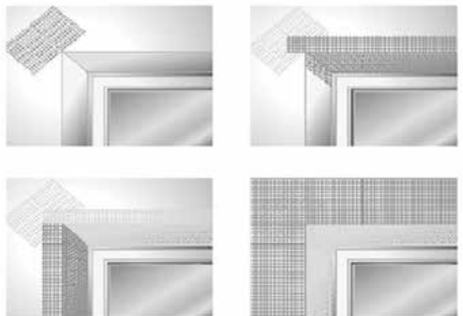
Figura 103 - Esquema de aplicação de rede para reforço dos ângulos nos vãos
