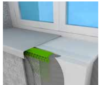
Figura 42 - Peitoril em alumínio lacado branco
