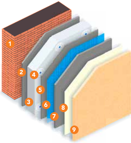
Figura 9 - Componentes do SISTEMA THERMINNOV
