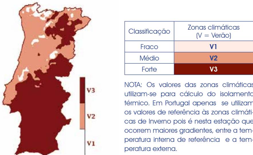
Figura 3 - Zonas climáticas de Portugal no verão
