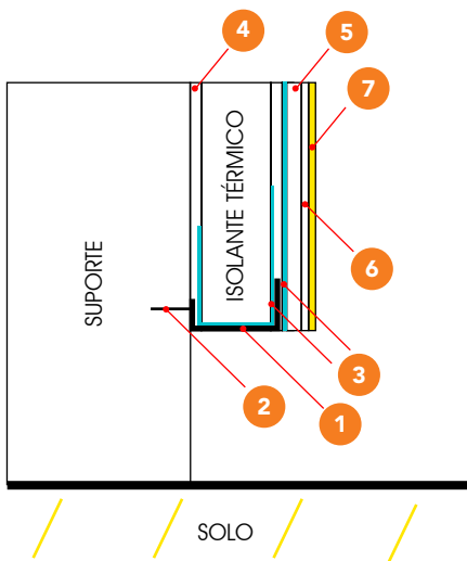
Figura 76 - Esquema de colocação do perfil de arranque.
