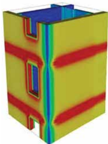
Figura 4 - Termografias
