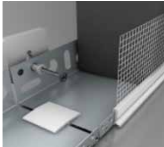
Figura 20 - Ligador de perfil de arranque
