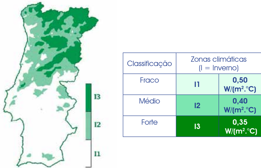
Figura 2 - Zonas climáticas de Portugal no inverno
